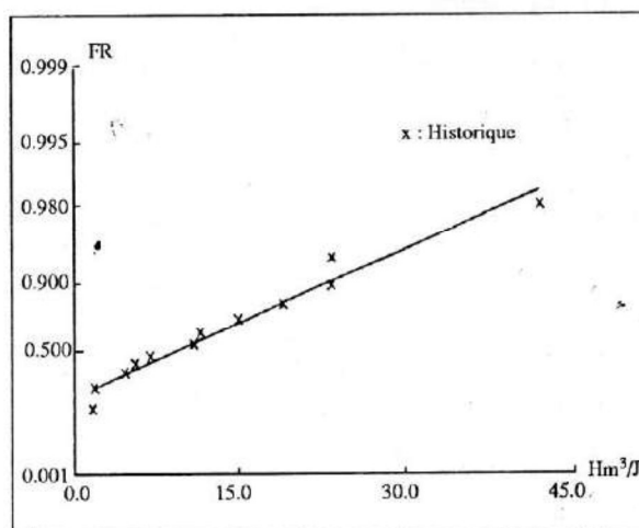
Figure 3 : Débits maxima journaliers (barrage Cheffia) 1978-1989.
