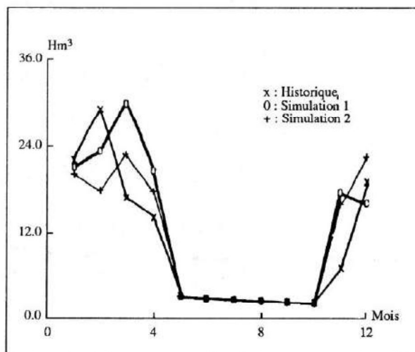
Figure 6 : Débits mensuels (barrage Cheffia) 1978-1989.
