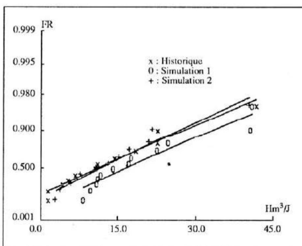
Figure 5 : Comparaison des débits maxima journaliers (barrage Cheffia) 1978-1989.
