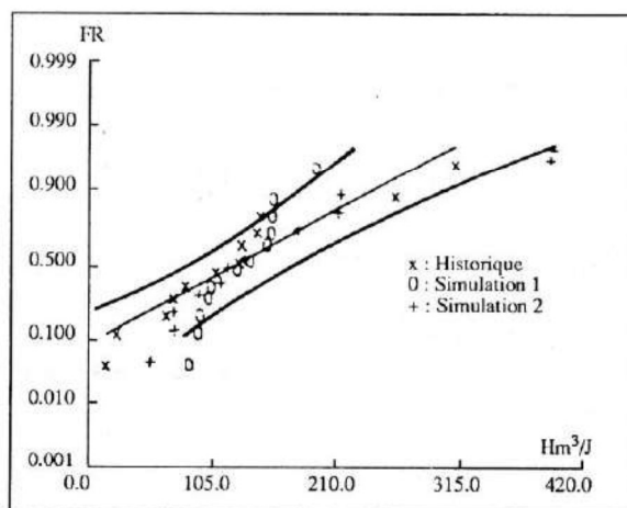
Figure 4 : Comparaison des débits annuels (barrage Cheffia) 1978-1989.
