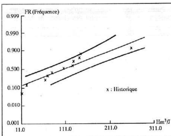
Figure 2 : Débits annuels (barrage Cheffia) 1978-1989.
