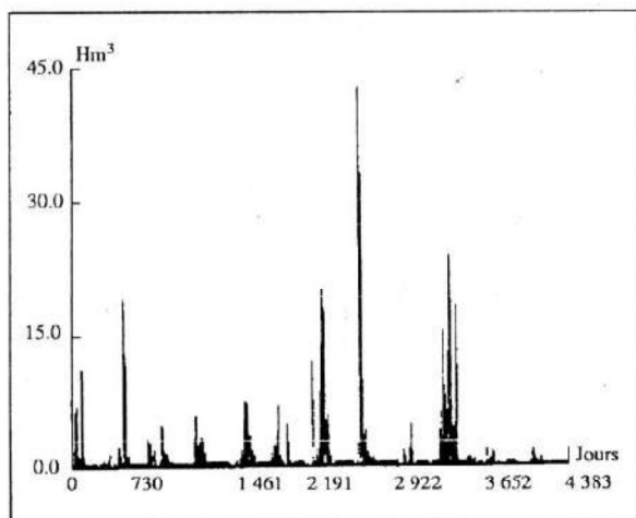
Figure 1 : Débits journaliers (barrage Cheffia).
